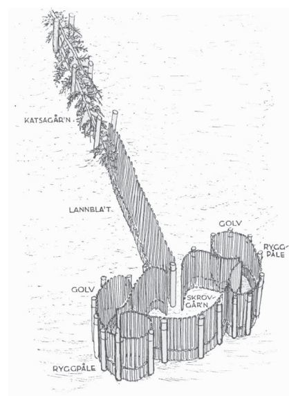
Figur 2. Illustration av hur en katsa ska uppföras. "Katsagår'n" är den inre risarmen, "Lannblåt" är spjälmmattan och "Skrovgår'n" den yttre fångstgården. Ur Claesson 1937.
