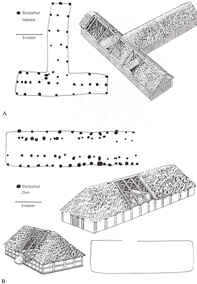
Fig.4. Överst (A) : En bondgård från 1200-talet i skiftesverk. Pebringe på Själland. Efter N.K. Liebgott 1984. - Underst (B) : Utvecklingen från jordgrävda stolpar till korsvirke påstensyll under 1300-talet. Hejninge på Själland. Efter N.K. Liebgott 1984.
