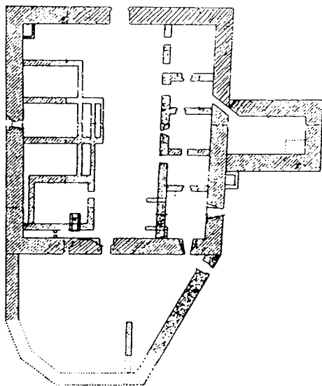
Miklaborg på Ragnhildsholmen vid Kungahälla.
