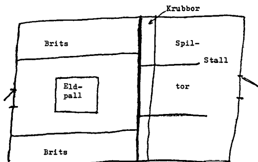
Fig 3. Överst "Timmerkoja med sammanbyggt stall" Ill. från Eriksson 1976:52. Den nedre bilden visar en timmerkoja från Vilhelmina sn, Lappland, omkr. 1896. "Avdelningen för folket var 6x6 m och stallet var 3x6 m." Ill. från EU 40 421:350.
